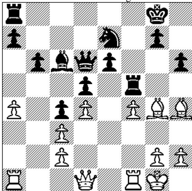
Diagram na 18. L94
